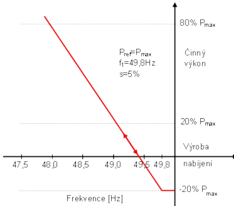
Obr. 18 Ilustrativní znázornění frekvenční odezvy činného výkonu na podfrekvenci u akumulačního zařízení.
